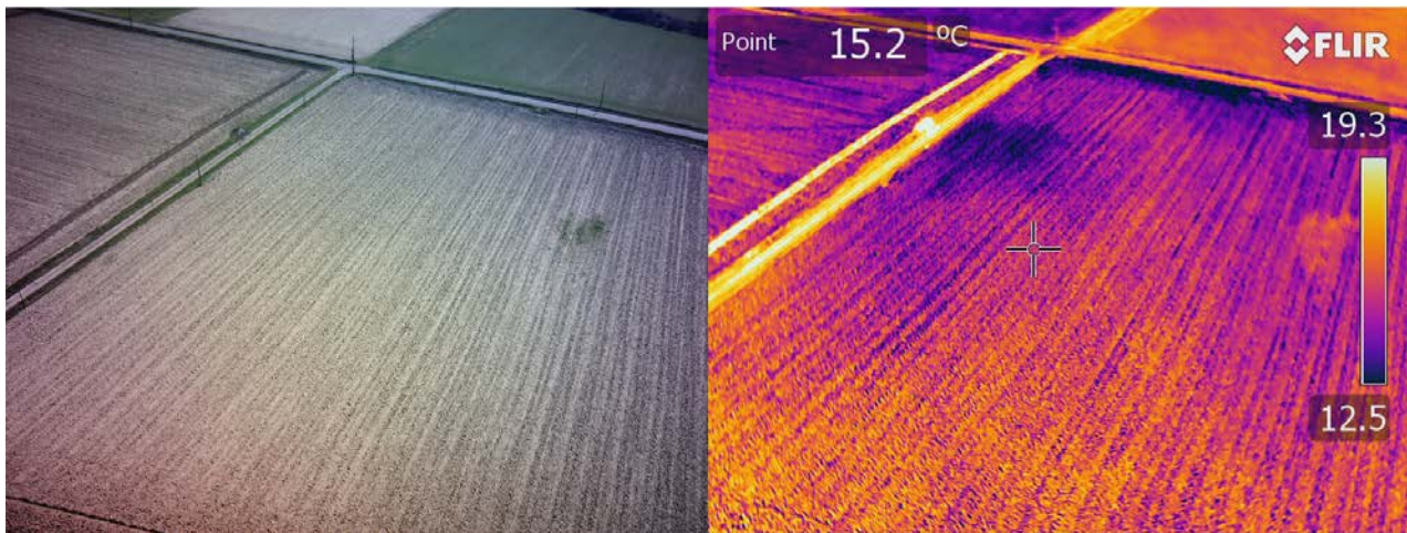
Figure 4 : Thermographie sur sol nu à Saint-Porquier (82). Aucune anomalie n'est visible sur la photographie classique (à gauche) alors qu'une anomalie froide est visible dans le coin supérieur gauche de la parcelle (à droite) correspondant à l'emprise d'un site archéologique repéré en prospection au sol.
